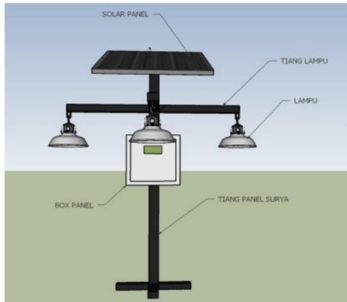
Gambar 2. Gambar Desain Simulasi Alat
