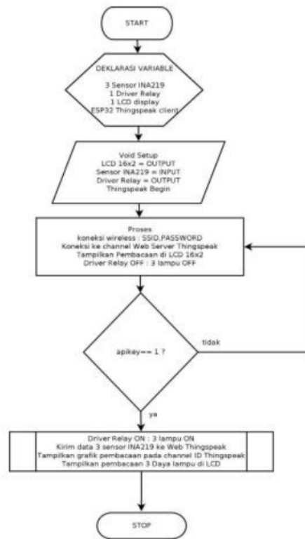
Gambar 6. Flowchart Sistem Keseluruhan
