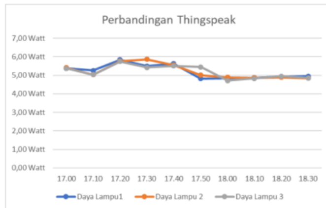
Gambar 10. Grafik Pengujian Daya Beban Lampu pada Thingspeak
