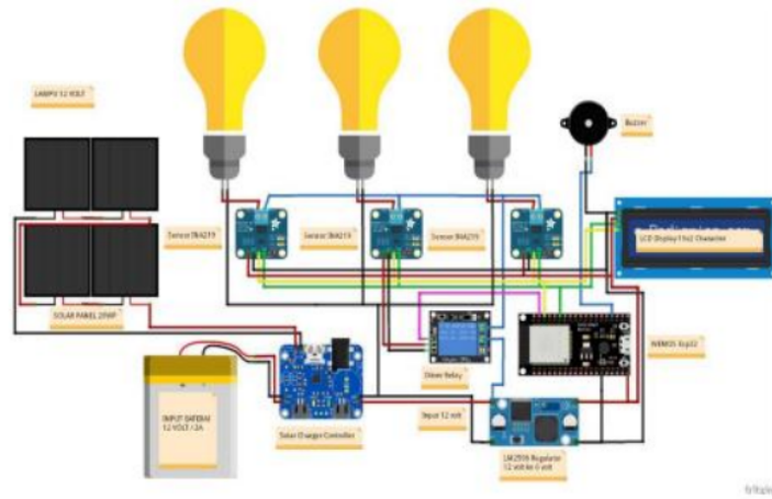
Gambar 4. Wiring Diagram Sistem Utama
