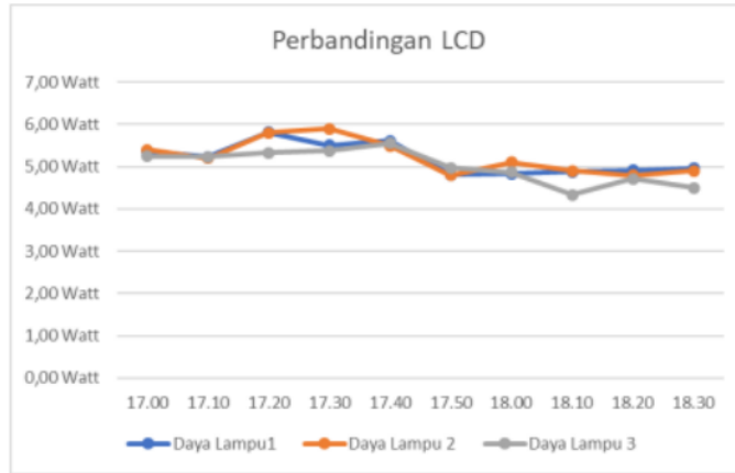
Gambar 9. Grafik Pengujian Daya Beban Lampu pada LCD
