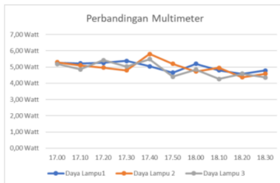
Gambar 8. Grafik Pengujian Daya Lampu pada Multimeter Digital
