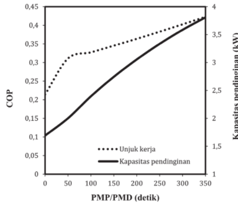
Gambar 5. Pengaruh Waktu Pemulihan Masa Pada COP dan Kapasitas Pendinginan. Sumber (Penulis, 2022)
