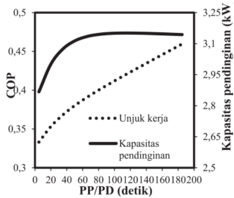
Gambar 4. Pengaruh Waktu Pra-pemanasan dan Pra-pendinginan terhadap COP dan kapasitas pendinginan. Sumber (Penulis, 2022)
