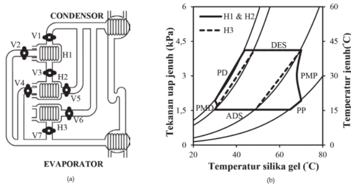
Gambar 1. Skematika Sistem Pendingin Adsorpsi Dengan Pemanasan Ulang Kombinasi (a) dan Diagram Temperatur-Tekanan-Konsentrasi (PTK) (b) Sumber (Penulis, 2022)
