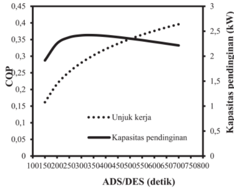
Gambar 3. Pengaruh Waktu Adsorpsi / Desorpsi terhadap Unjuk kerja dan kapasitas pendinginan Sumber (Penulis, 2022)
