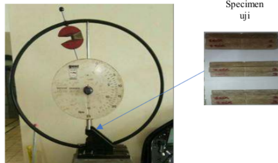
Gambar 3. Alat pengujian impact
