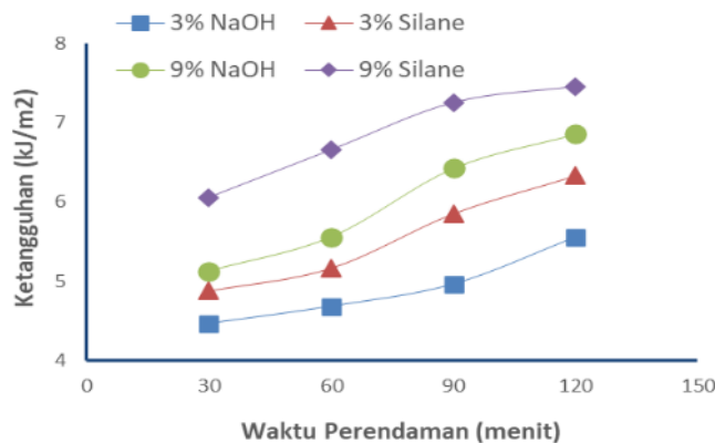
Gambar 5. Hubungan antara waktu perendaman dengan ketangguhan
