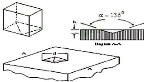
Gambar 2. Skema pengujian kekerasan
