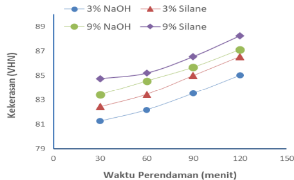
Gambar 4. Hubungan antara waktu perendaman dengan kekerasan
