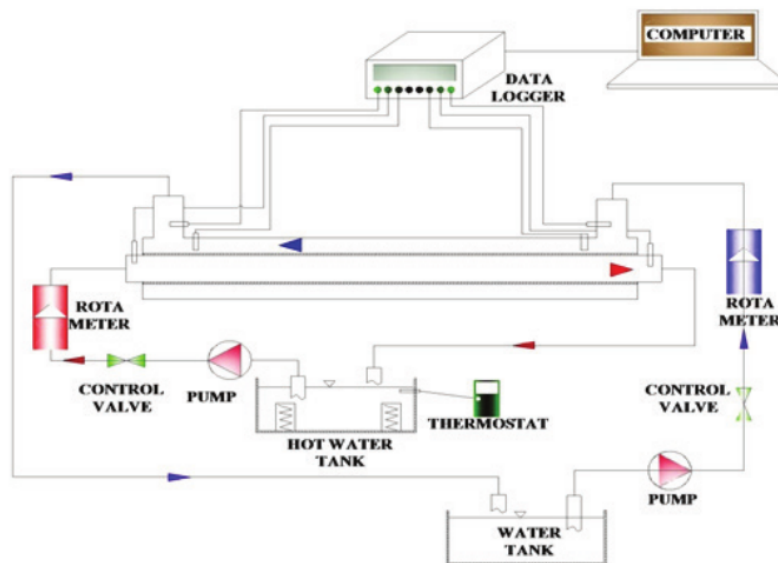
Gambar 3. Skema experiment apparatus Sumber: Sunu P.W dan Rasta I M. (2017)
