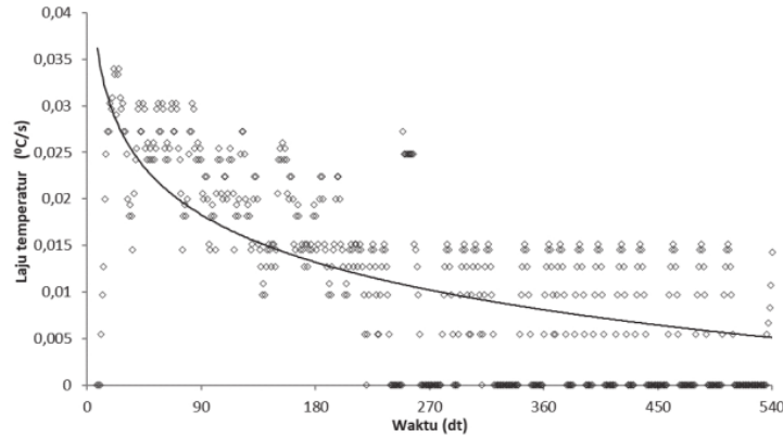
Gambar 7. Laju peningkatan temperatur fluida dingin pada groove 2 mm Sumber: Dokumentasi pribadi
