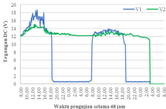
Gambar 3. Tegangan luaran sel-PV dan baterai
