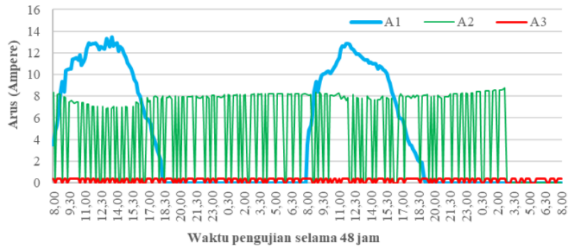
Gambar 4. Nilai arus luaran sel PV, baterai dan yang digunakan sistem refrigerasi
