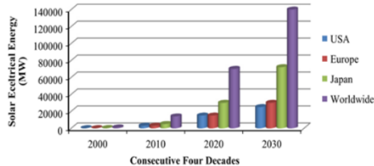
Gambar 1. Produksi energi listrik tenaga surya global berbasis PV selama empat dekade
