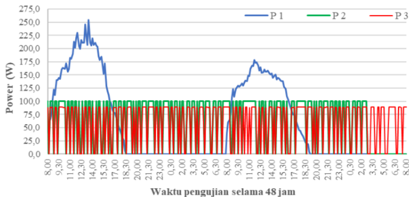
Gambar 5. Daya yang dihasilkan sel-PV, disimpan baterai dan digunakan sistem refrigerasi
