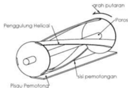
Gambar 1 Mekanisme Penggulung Dalam Rancangan Pemotong Rumput Mini
