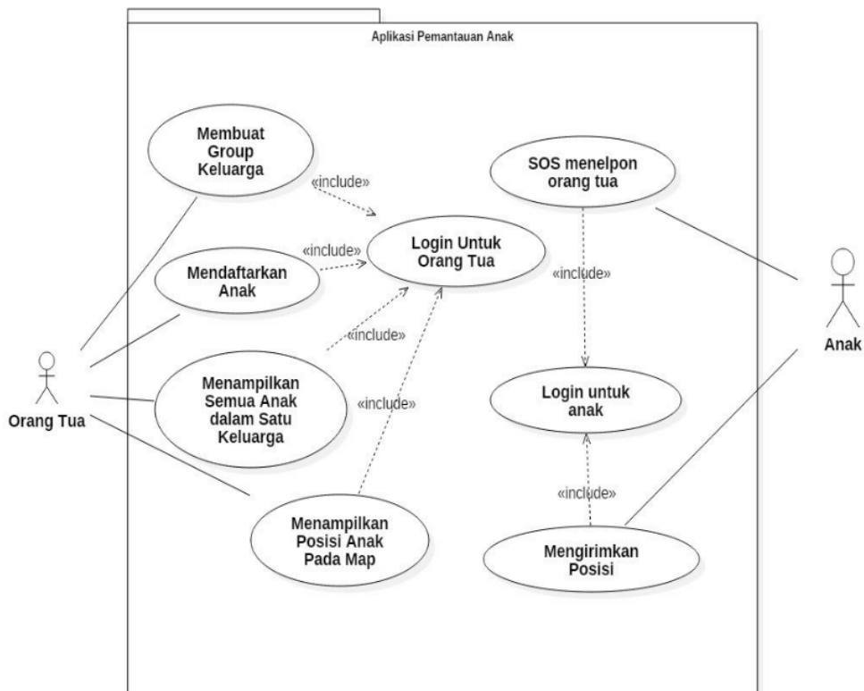
Gambar 3. Gambar Use Case Aplikasi Pemantauan Posisi Anak
