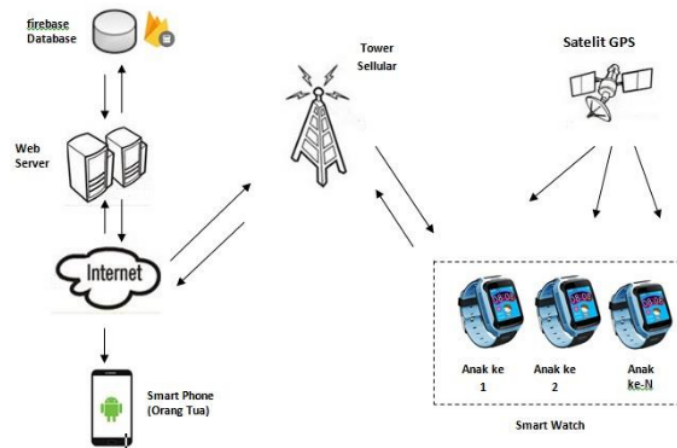
Gambar 1. Arsitektur Perangkat Lunak Pemantauan Posisi Anak
