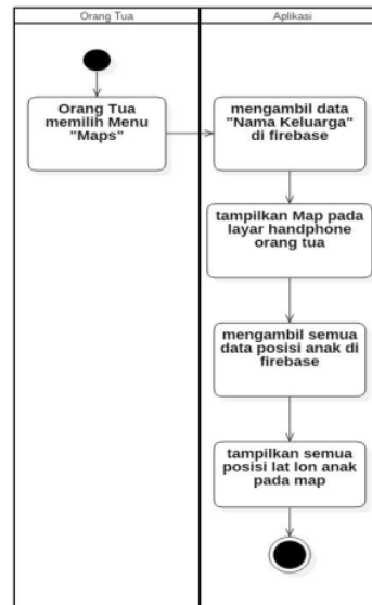
Gambar 8. Activity Diagram Menampilkan Posisi Anak Pada Map
