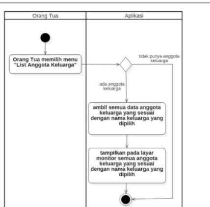
Gambar 7. Activity Diagram Menampilkan Anak Dalam Satu Keluarga
