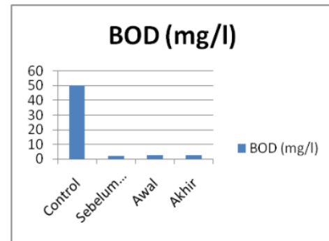
Gambar 4.2 Perbandingan nilai BOD_5 air limbah sebelum dan setelah pengolahan
