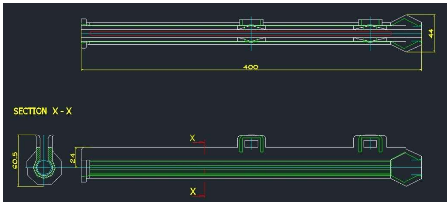
Gambar 14 Dimensi Tekep Belokan Extension
