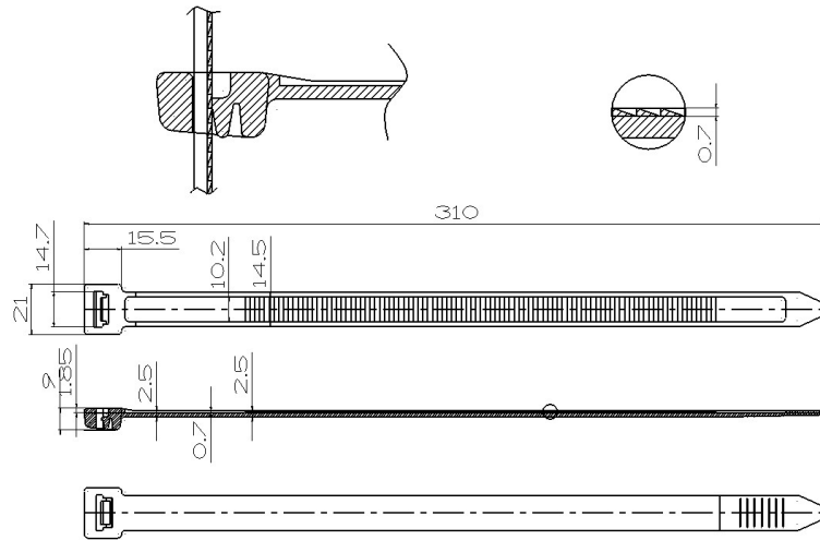
Gambar 15 Dimensi Sabuk Pendek
