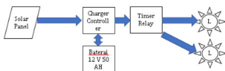
Gb. 5 Sistem PLTS untuk Penerangan Kolam Pembesaran Ikan
