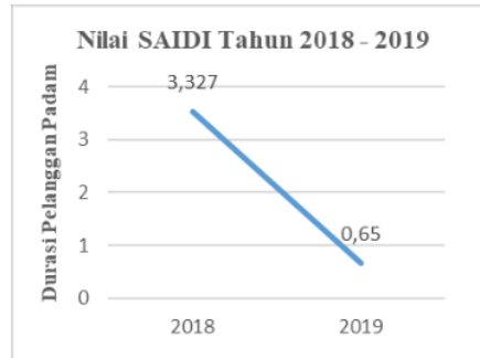
Gambar 1. Grafik Perbandingan Nilai SAIDI
