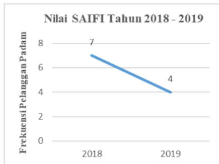
Gambar 2. Grafik Perbandingan Nilai SAIFI
