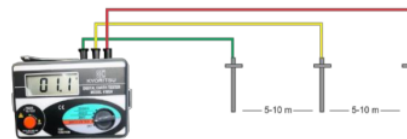
Gambar 2 Rangkaian pengukuran tahanan pentanahan gardu.
