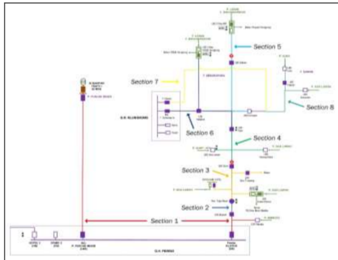
Gambar 1. Pembagian section Penyulang Puncak Mundi
