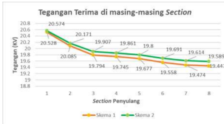
Gambar 2. Grafik tegangan terima di masing-masing section
