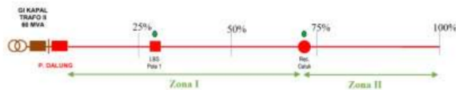
Gambar 1. Jaringan Penyulang Dalung
