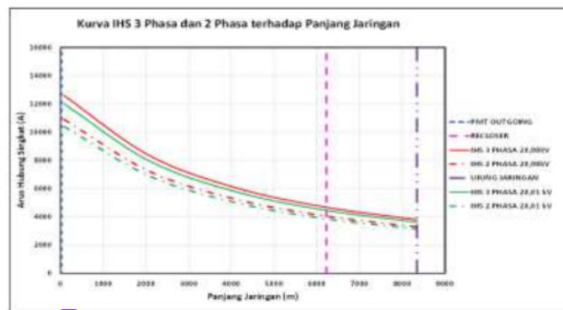
Gambar 3. Kurva Arus Gangguan Hubung Singkat 3 dan 2 Fasa Penyulang Dalung
