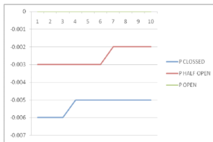
Grafik 1. Tekanan sisi atas
