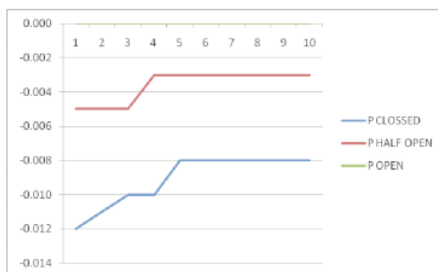
Grafik 3. Tekanan sisi bawah
