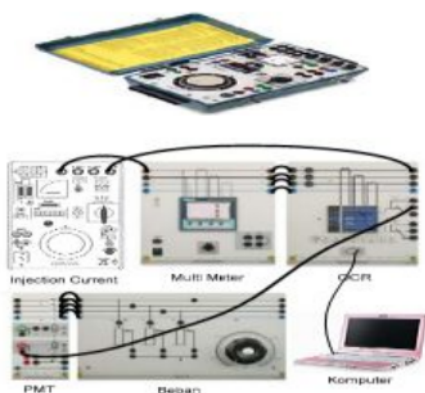
Gambar.9. Rangkaian uji relay arus lebih SPAJ 131 C
