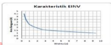
1 Gambar 12. Karakteristik waktu Extremely Inverse
