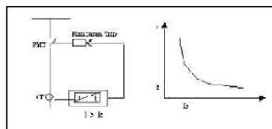
Gambar.5. Karakteristik Tripping Relay Arus LebihWaktu Inverse
