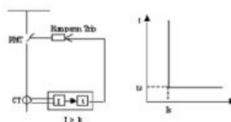
Gambar.4. Karakteristik Tripping Relay Arus Lebih Waktu Definite
