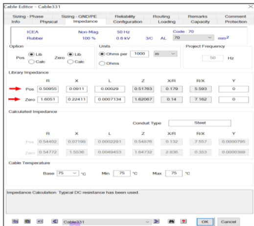
Gambar 7. Input data pengantar pada ETAP 16.00
