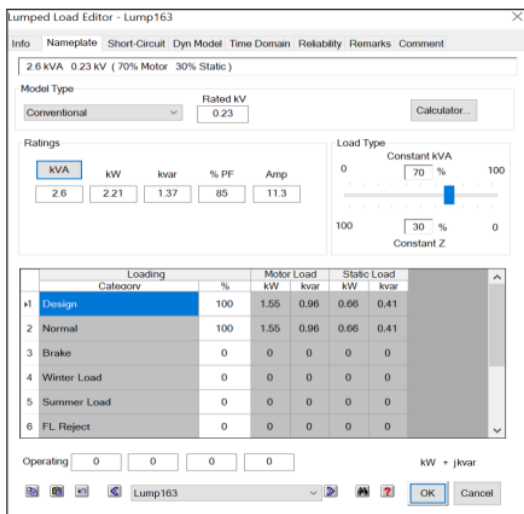
Gambar 8. Input data beban pada ETAP 16.00
