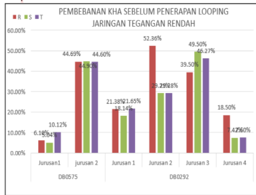
Gambar 12. Diagram batang pembebanan kha sebelum penerapan looping JTR
