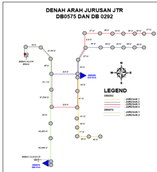
Gambar 9. Denah arah jurusan jaringan tegangan rendah
