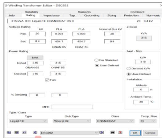
Gambar 6. Input data transformator pada ETAP 16.00
