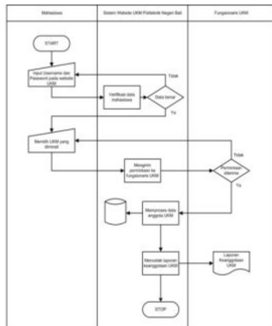
Gambar 3. Pendaftaran anggota UKM secara daring.
