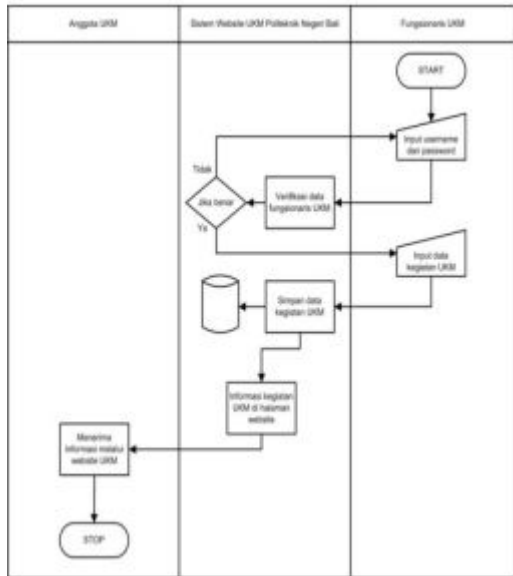
Gambar 4. Penyampaian informasi secara Daring
