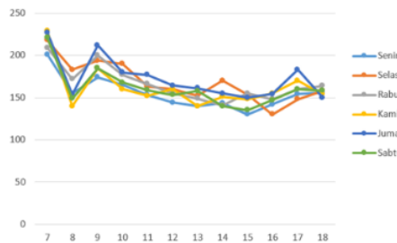
Gambar 6. Daya Luar Panel Surya
