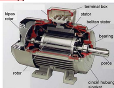
Gambar 1. Konstruksi Motor Induksi 3 fasa
