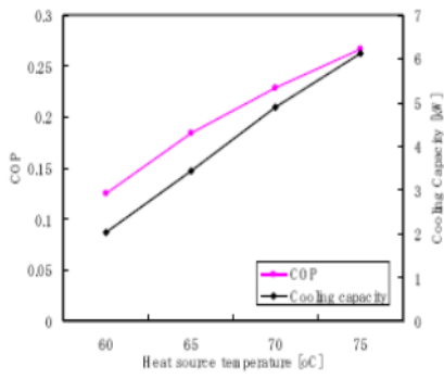
Gambar 3. Pengaruh temperatur pemanasan terhadap unjuk kerja mesin
