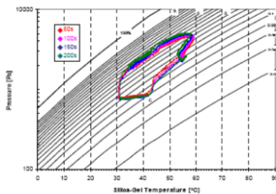
Gambar 6. Pengaruh waktu mass recovery pada Duhimg Diagram
