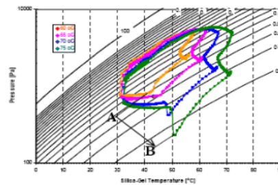
Gambar 4. Pengaruh temperatur pemanasan pada Duhring Diagram.
