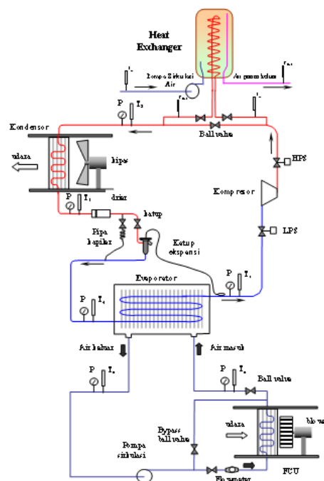
Gambar 1. Diagram Skematik Perangkat Pengujian AC Jenis Water Chiller.
