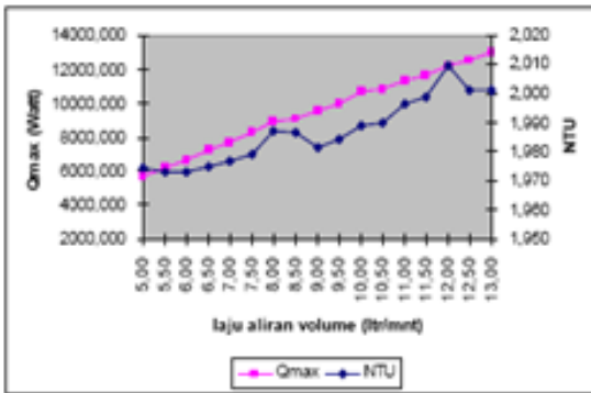
Gambar 3. Grafik Hubungan NTU, Temperatur dan Laju Aliran Volume
