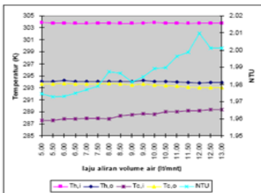
Gambar 4. Grafik Hubungan NTU, Qmax Terhadap Laju Aliran Volume.
