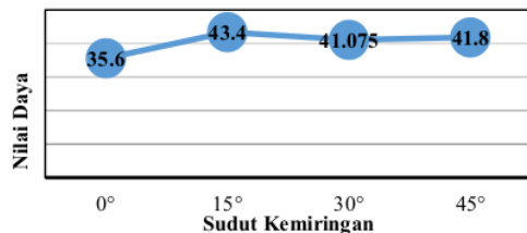
Gambar 6. Grafik daya maksimum pada semua sudut
