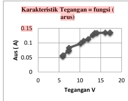
Gambar 8. karakteristik Tegangan = fungsi ( arus)
