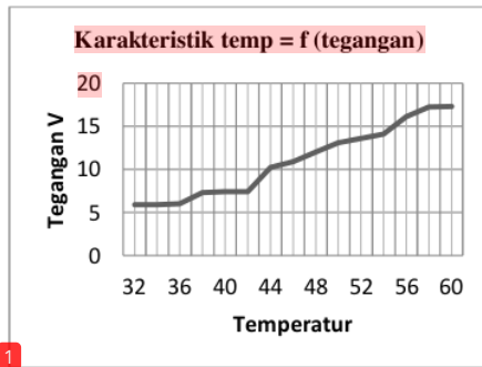
Gambar 6. Karakteristik Temperatur Pv = f tegangan ( V) pada beban 200 ohm
