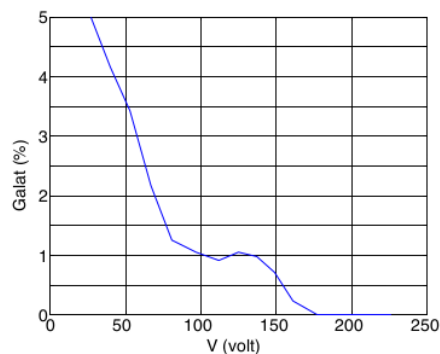
Gambar 6. Kesalahan Pengukuran Tegangan RMS Jala-jala
