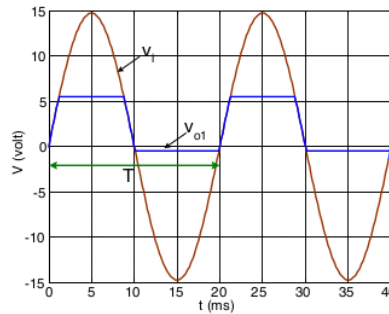
Gambar 2. Sinyal Input Mikrokontroler
