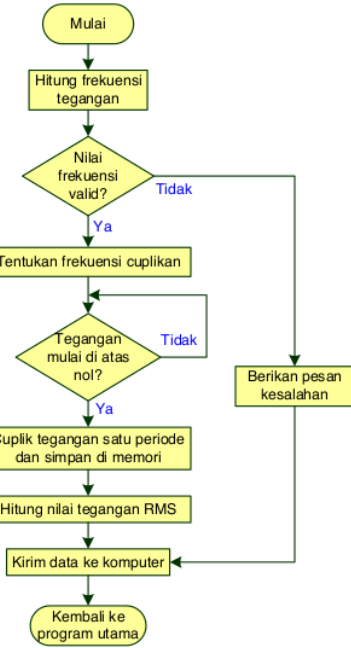
Gambar 3. Diagram Alir Simulasi
