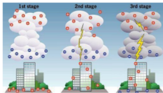
Gambar 1. Proses ionisasi terjadinya petir [8].
