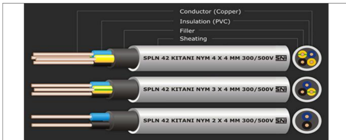
Gambar 5. Kabel NYM
