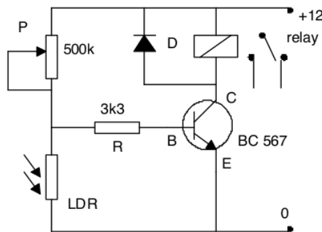
Gambar 2. Rangkaian sensor LDR
